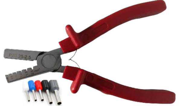
İZOLELİ, İZOLESİZ YÜKSÜK SIKMA PENSESİ 0,50 - 2,5 mm 2
